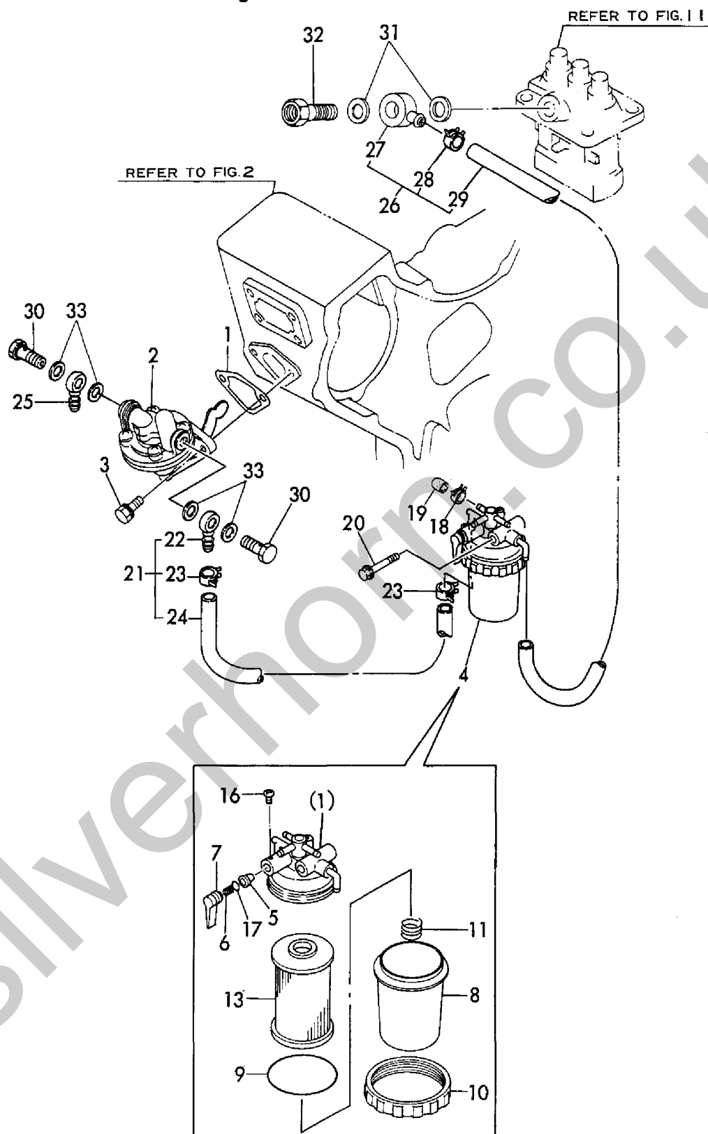
Fig. 12 燃料パイプ FUEL PIPE
