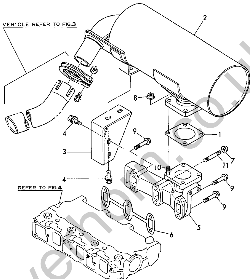
Fig. 6 排気マニホールド&サイレンサ EXHAUST MANIFOLD & SILENCER
