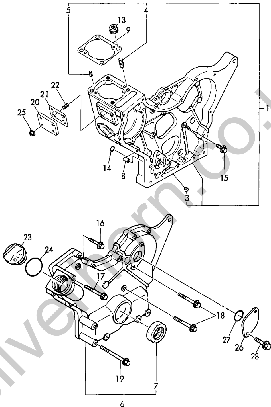
Fig. 2 ギヤケース GEAR HOUSING
