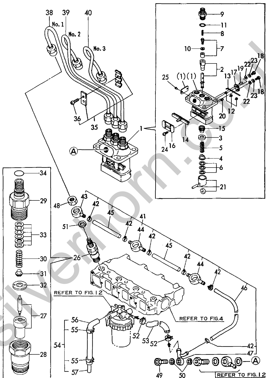
Fig. 11 燃料噴射装置 FUEL INJECTION DEVICE
