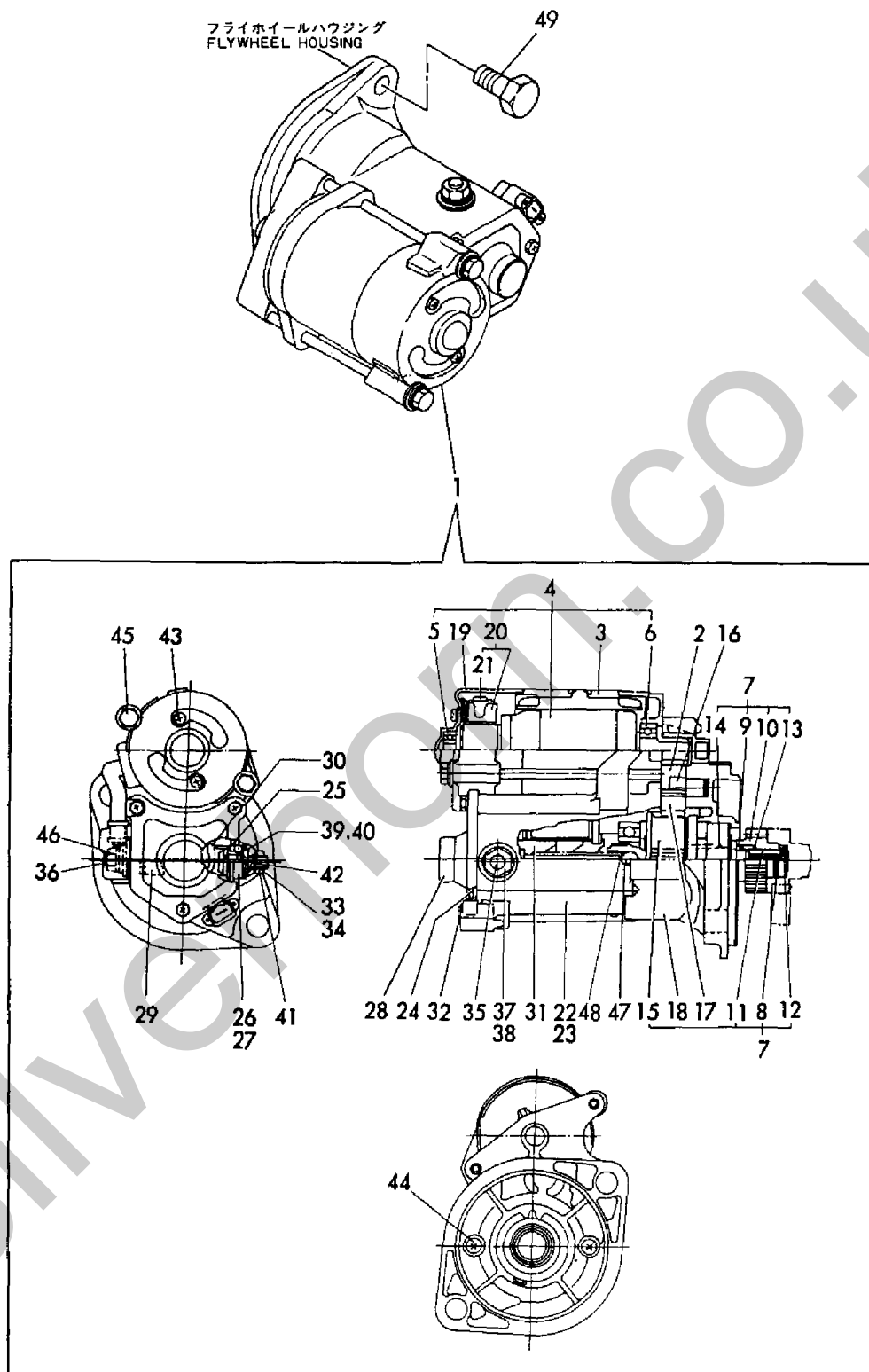
Fig. 14 スターティングモータ STARTING MOTOR
